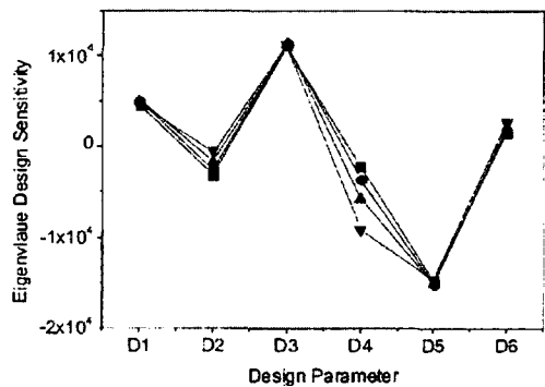
(d) Fourth eigenvalue
